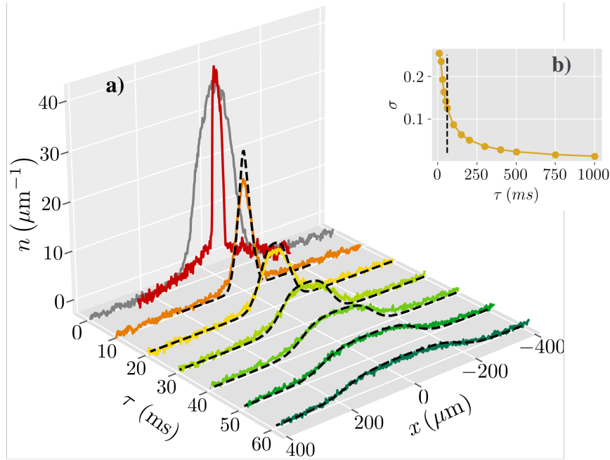
FIGURE V .8 – (a) La tranche , centrée en x_0 = 0 \mu\text{m} , subit une expansion le long de l’axe longitudinal et d’une largeur \ell = 37 \mu\text{m} . Le profil initial du gaz est montré en gris. Les variations de densité pour différents temps d’expansion sont représentées par des courbes colorées. Les lignes pointillées noires indiquent les résultats des simulations GHD pour une distribution de rapidités initialement thermique, paramétrée par la température T et le potentiel chimique \mu(x_0) = \mu , tels qu’ils sont extraits du profil de densité in situ. (b) L’écart-type \sigma(\tau) (eq. (V .34)) est calculé entre la distribution de rapidités et les résultats des simulations GHD en fonction du temps d’expansion \tau . La ligne verticale noire correspond au temps d’expansion utilisé dans l’expérience.
